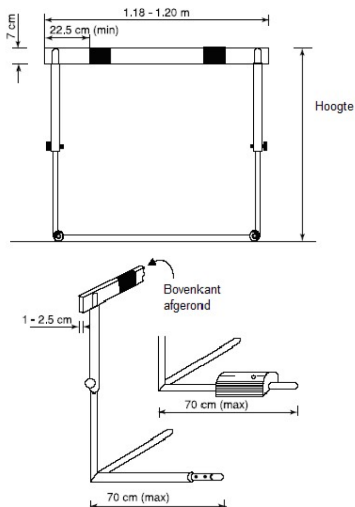
Afbeelding TR22 – Voorbeeld van een horde
