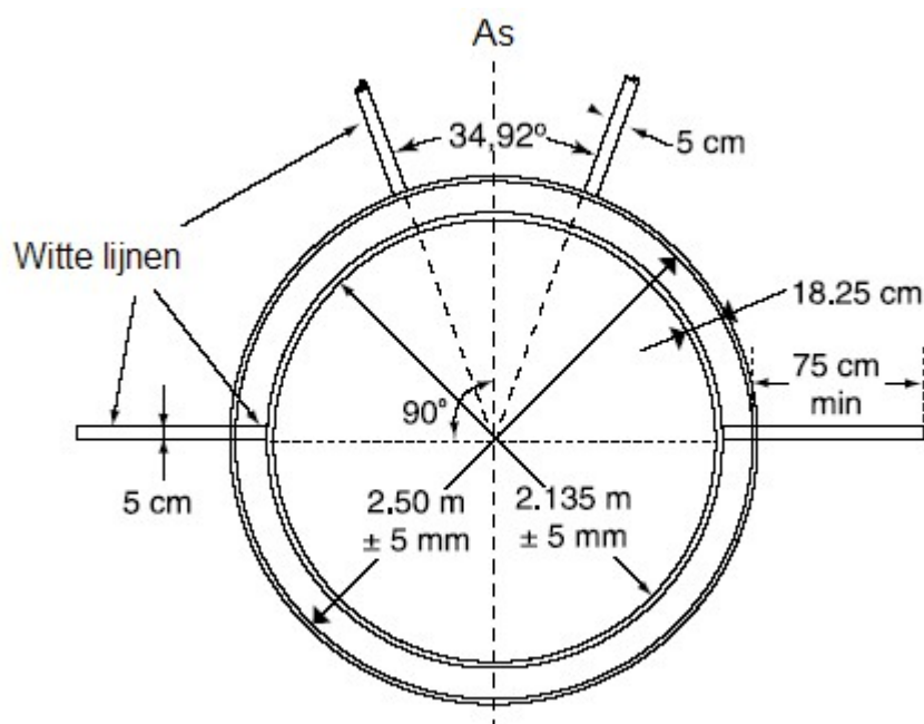
Afbeelding (c) TR32 – Werp cirkel voor Hamerslingeren
