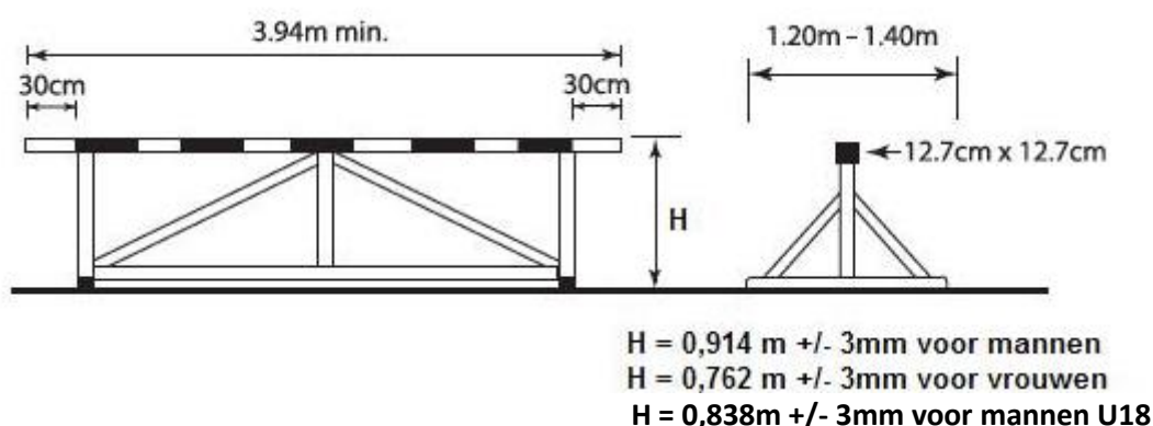
Afbeelding (a) TR23 – Voorbeeld van een steeplebalk
