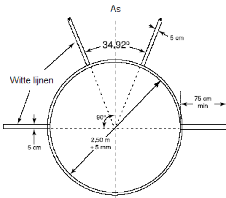
Afbeelding (b) TR32 – Wercirkel voor Discuswerpen
