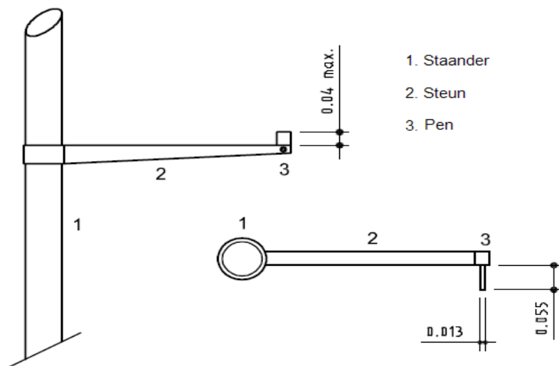
Afbeelding (b) TR28 - Staanders voor de lat bij het polsstokspringen (zicht vanaf de landingsplaats en bovenaanzicht)
