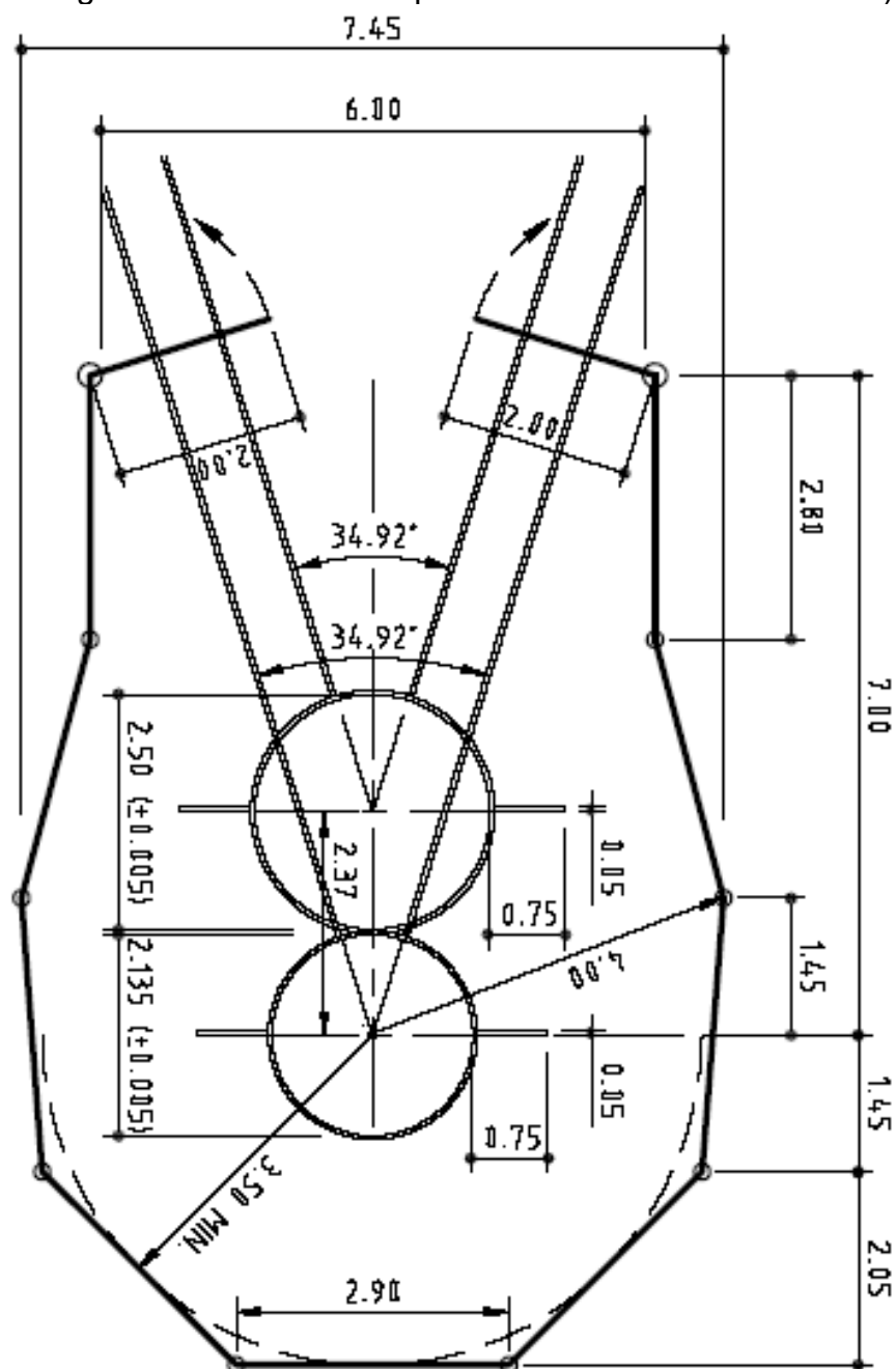
Afbeelding (c) TR37 – Kooi voor Hamerslingeren en Discuswerpen met afzonderlijke werpcirkels
