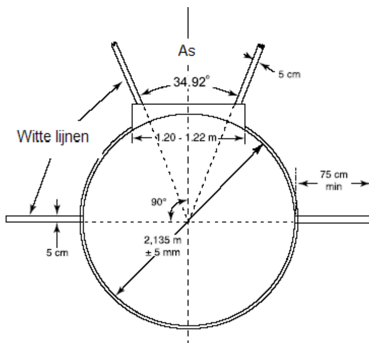
Afbeelding (a) TR32 – Wercirkel voor Kogelstoten
